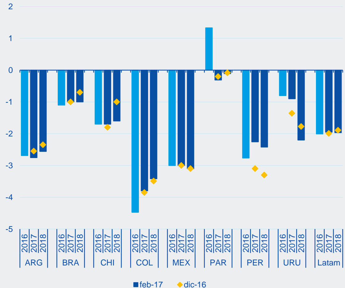
LATAM: DÉFICIT POR CUENTA CORRIENTE (%PIB)
